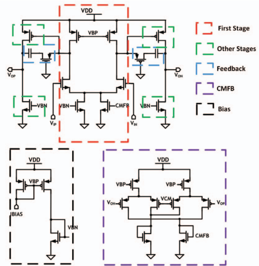
Fig. 3: Subcircuits of OTA3.
